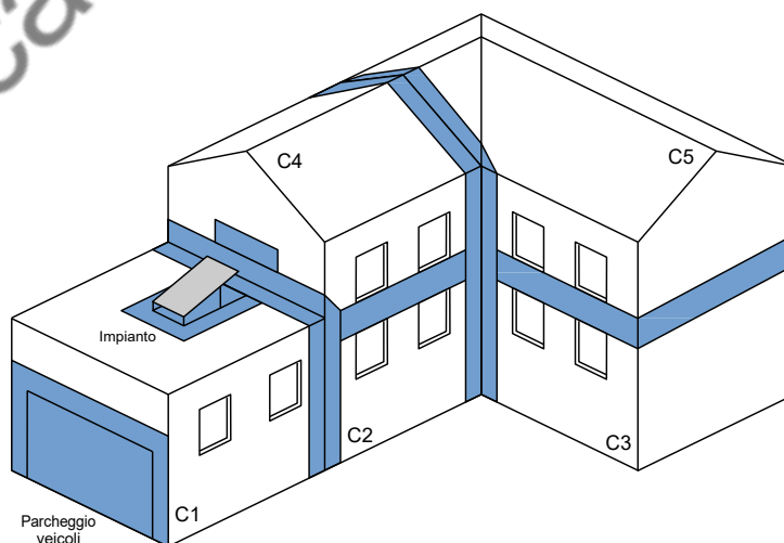
Illustrazione V.14-1: Esempio di fasce di separazione e protezioni per impianti e combustibili
