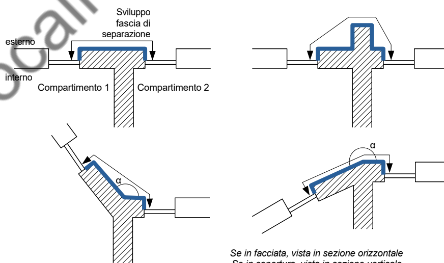
Illustrazione V.14-3: Esempi di fascia di separazione verticale in facciata o in copertura
