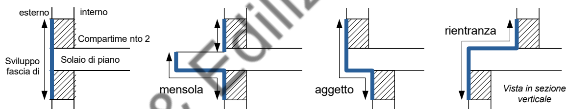
Illustrazione V.14-2: Esempi di fascia di separazione orizzontale in facciata
