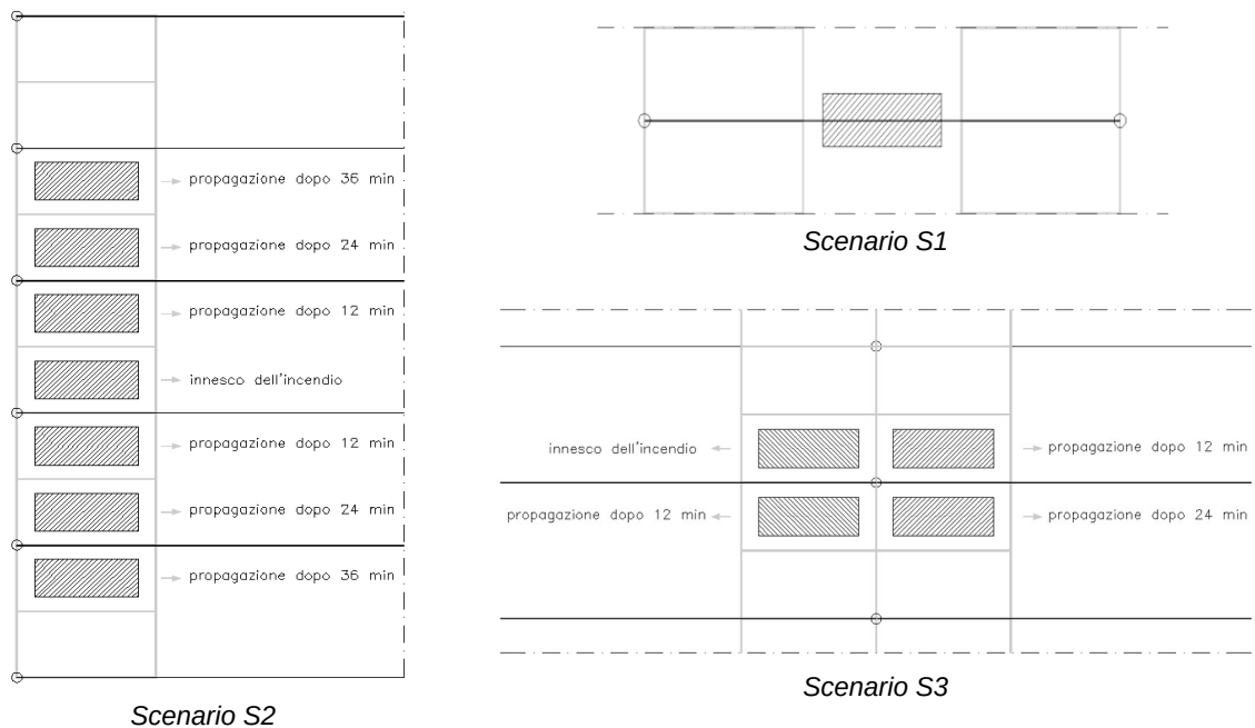
Illustrazione V.6-1: Schematizzazione degli scenari di incendio di progetto
