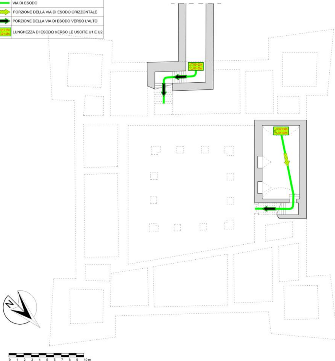
SISTEMA D'ESODO PIANO INTERRATO
