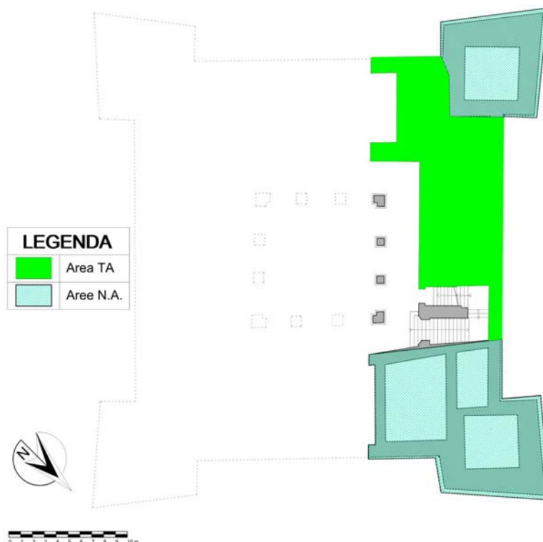
PLANIMETRIA PIANO INTERMEDIO - CLASSIFICAZIONE DELLE AREE
