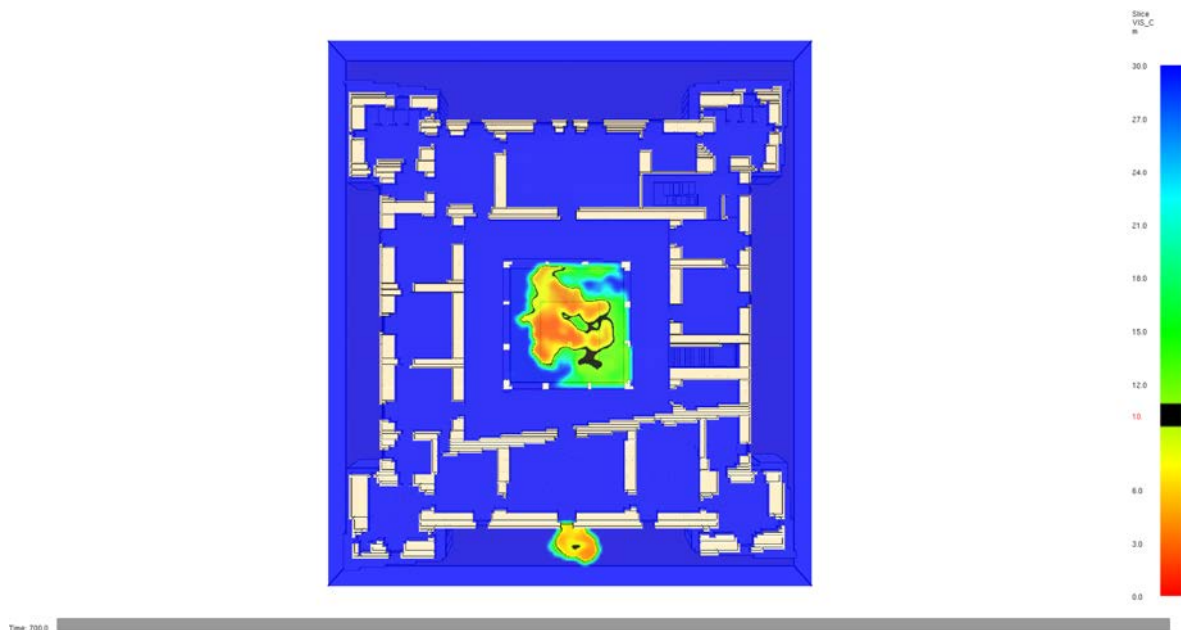
PROPAGAZIONE DEI FUMI AL PIANO PRIMO – VISIBILITÀ ( z = 1,80 m rispetto al piano calpestio) SCENARIO 2 – SENFC PRESENTE – Tempo di simulazione: 700 \text{ s} > \text{RSET} + t_{\text{marg}}
