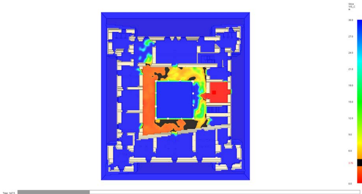
PROPAGAZIONE DEI FUMI AL PIANO PRIMO – VISIBILITÀ ( z = 1,80 m rispetto al piano calpestio) SCENARIO 1 – SENFC NON PRESENTE – Tempo di simulazione: 148 s < RSET
