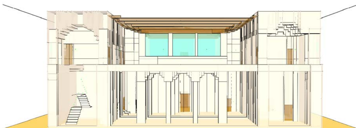
Sezione della zona scala 1 modellata con FDS
