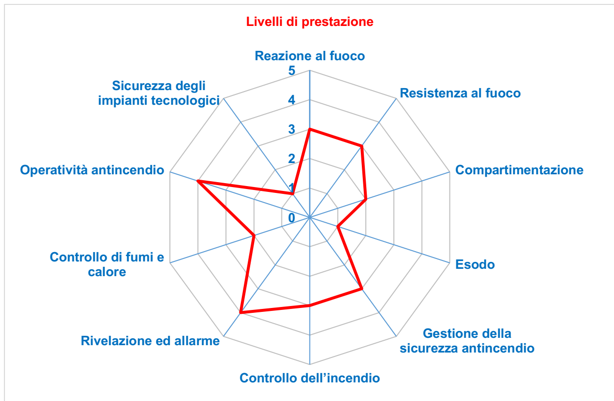
Rappresentazione polare dei I.P. Relativi alle misure costituenti la strategia antincendio
