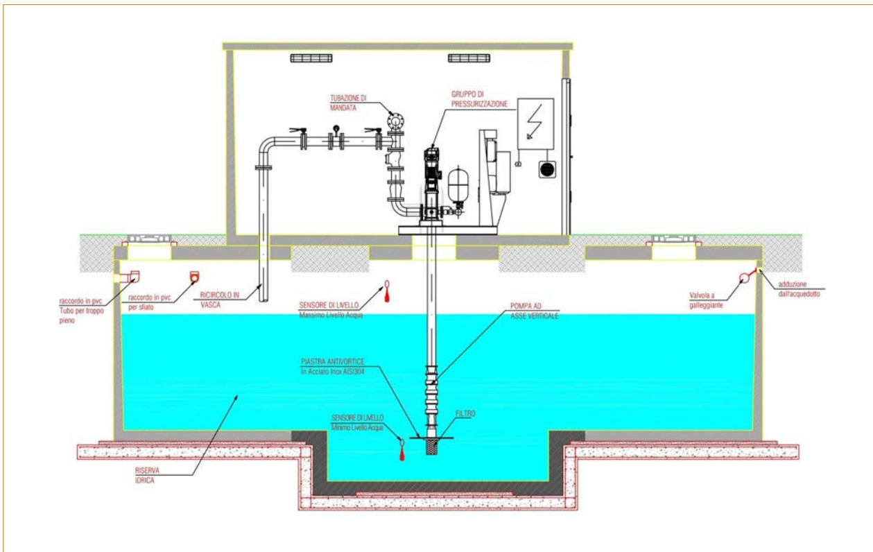
Esempio installazione impianto di pressurizzazione e riserva idrica - norma UNI 11292
