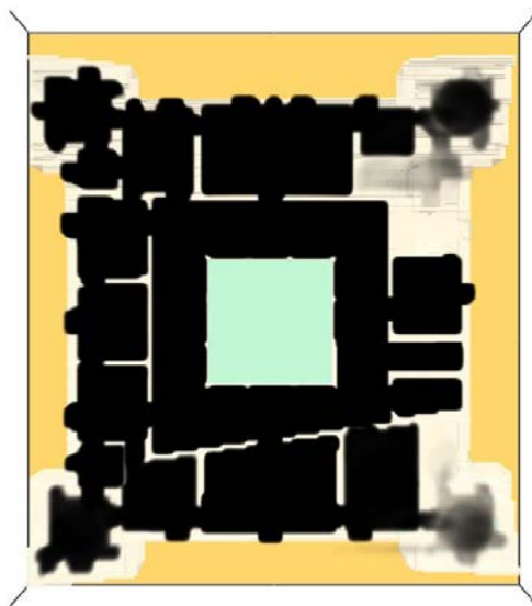
PROPAGAZIONE DEI FUMI AL PIANO PRIMO - SCENARIO 1 – SENFC NON PRESENTE Tempo di simulazione: 700 s > RSET + t_{\text{marg}}
