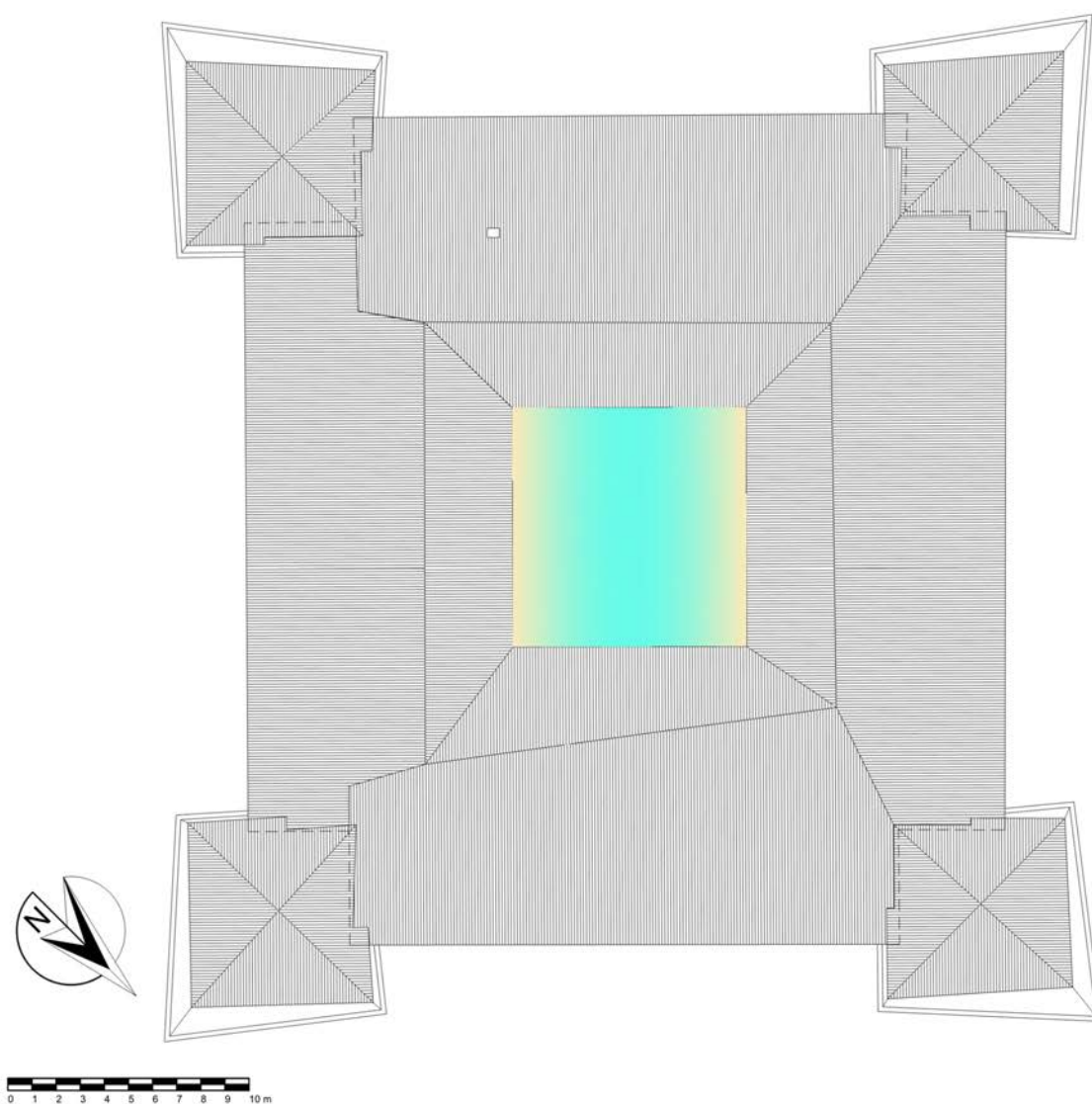
PLANIMETRIA COPERTURE
