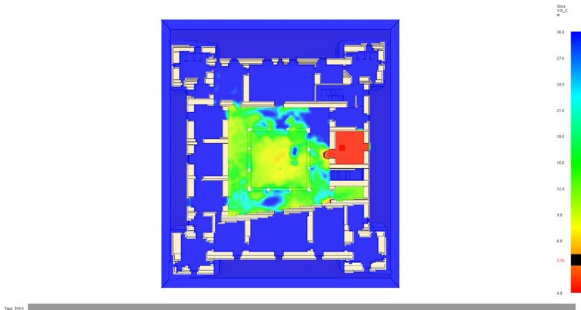
PROPAGAZIONE DEI FUMI AL PIANO PRIMO – VISIBILITÀ ( z = 1,80 m rispetto al piano calpestio) SCENARIO 1 – SENFC PRESENTE – Tempo di simulazione: 700 \text{ s} > RSET + t_{\text{marg}}
